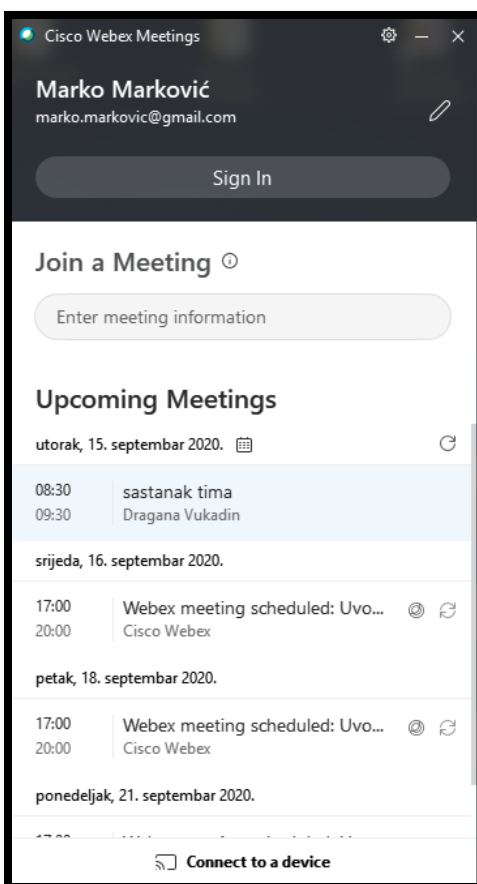
Slika 11 - Pokrenuta aplikacija
